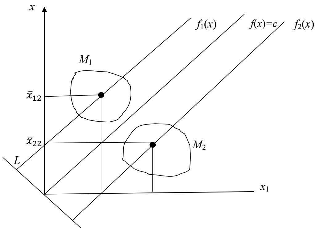
Рис. 3.2. Центри сукупностей, що класифікуються, та константа дискримінацій [133]
