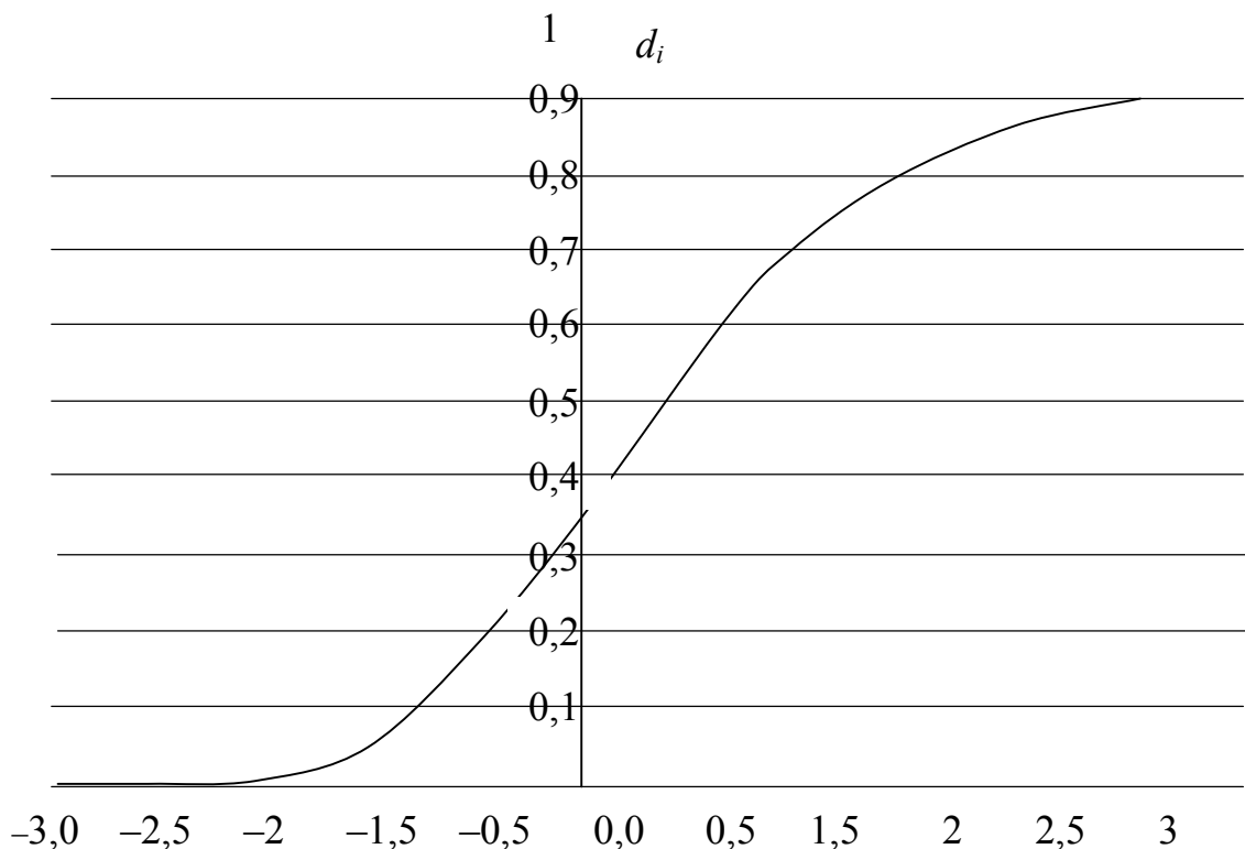
Рис. 3.3. Графік функції Харрінгтона
