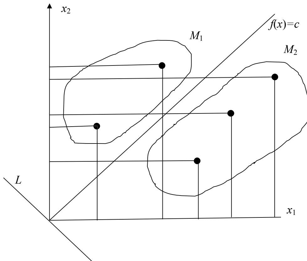
Рис. 3.1. Геометрична інтерпретація дискримінантної функції та дискримінантних змінних [133]
